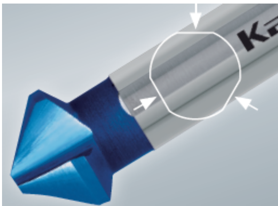
Każda średnica ma swój własny kąt przyłożenia.
