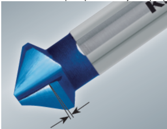
Relief regulowany promieniowo w zależności od średnicy - Kraweź skrawająca jest zawsze najwyższym punktem średnicy.
